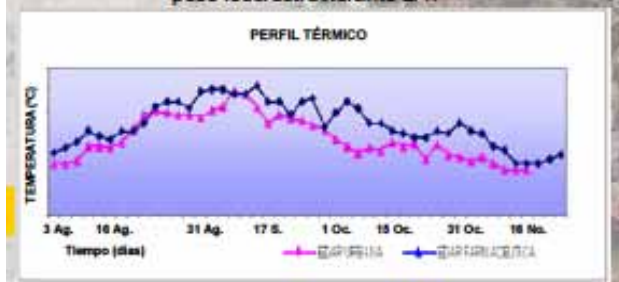
Figura 8. Perfil térmico del proceso.
